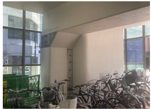
【第一通り駅耐震補強工事】
